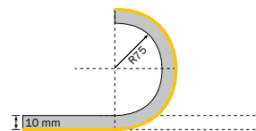
Biegeradius (Leuchtfläche aussen) bending radius (outer lighting area) rayon de courbure (lumineux extérieure)
