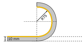
Biegeradius (Leuchtfläche innen) bending radius (inner lighting area) rayon de courbure (lumineux intérieure)
