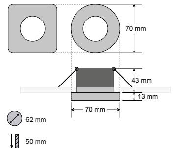
tuboquar L inkl. Vorschaltgerät (dimmbar) tuboquar L incl. ballast unit (dimmmable) tuboquar L avec ballast incl. (gradable)
