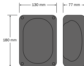
Multibox: B • S 30 • RC-Dim 30
