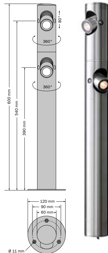
Montageflansch, Zubehör 93271 Mounting flange, accessory 93271 Bride de montage, accessoire 93271
